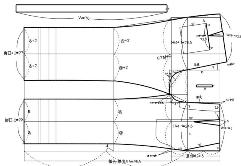
单褶单省男民族裤制图
