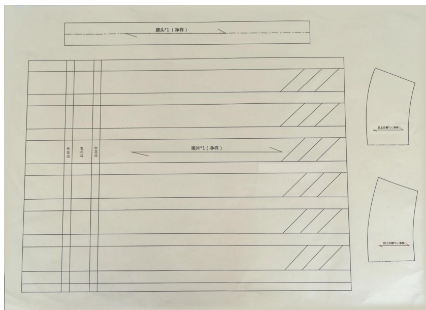
百褶裙制版——净样
