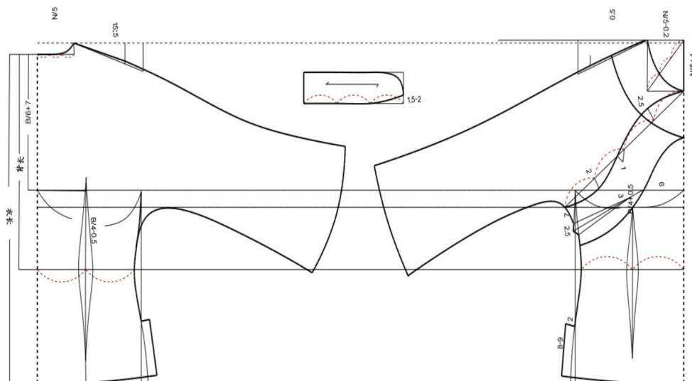
前片及部件制版
