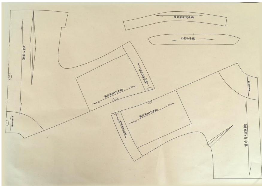
前右片、后片及领子净样
