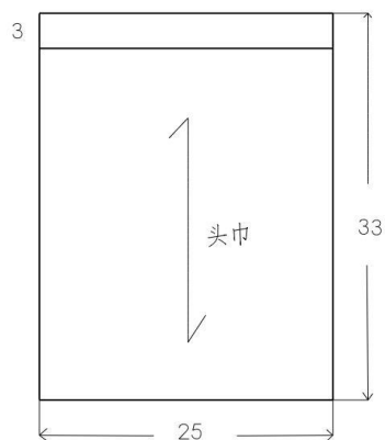
头巾制版图
